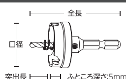
製品図
